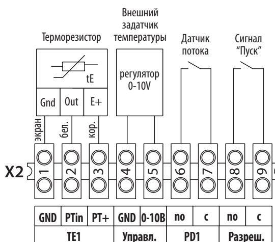
Схема внешних подключений
