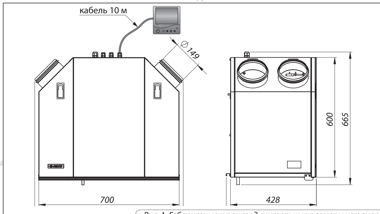
Рис. 1. Габаритные и присоединительные размеры установки
