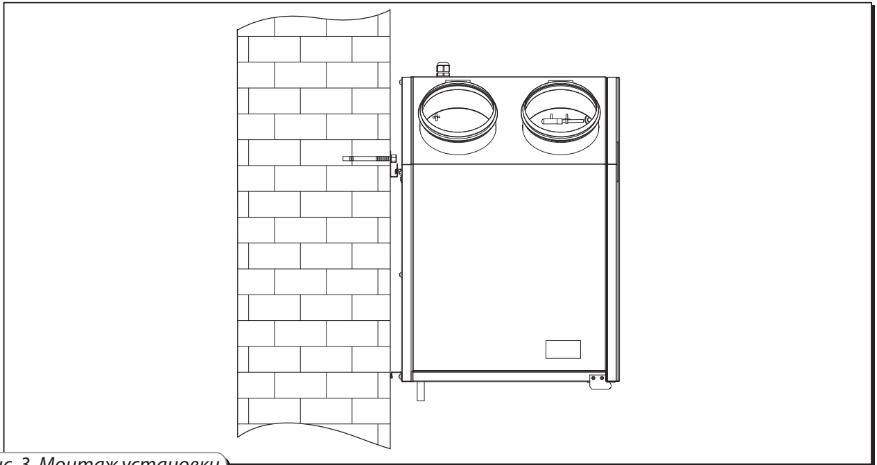
Рис. 3. Монтаж установки
