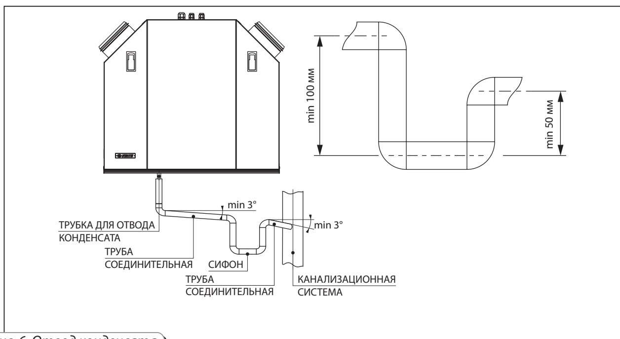
Рис. 6. Отвод конденсата
