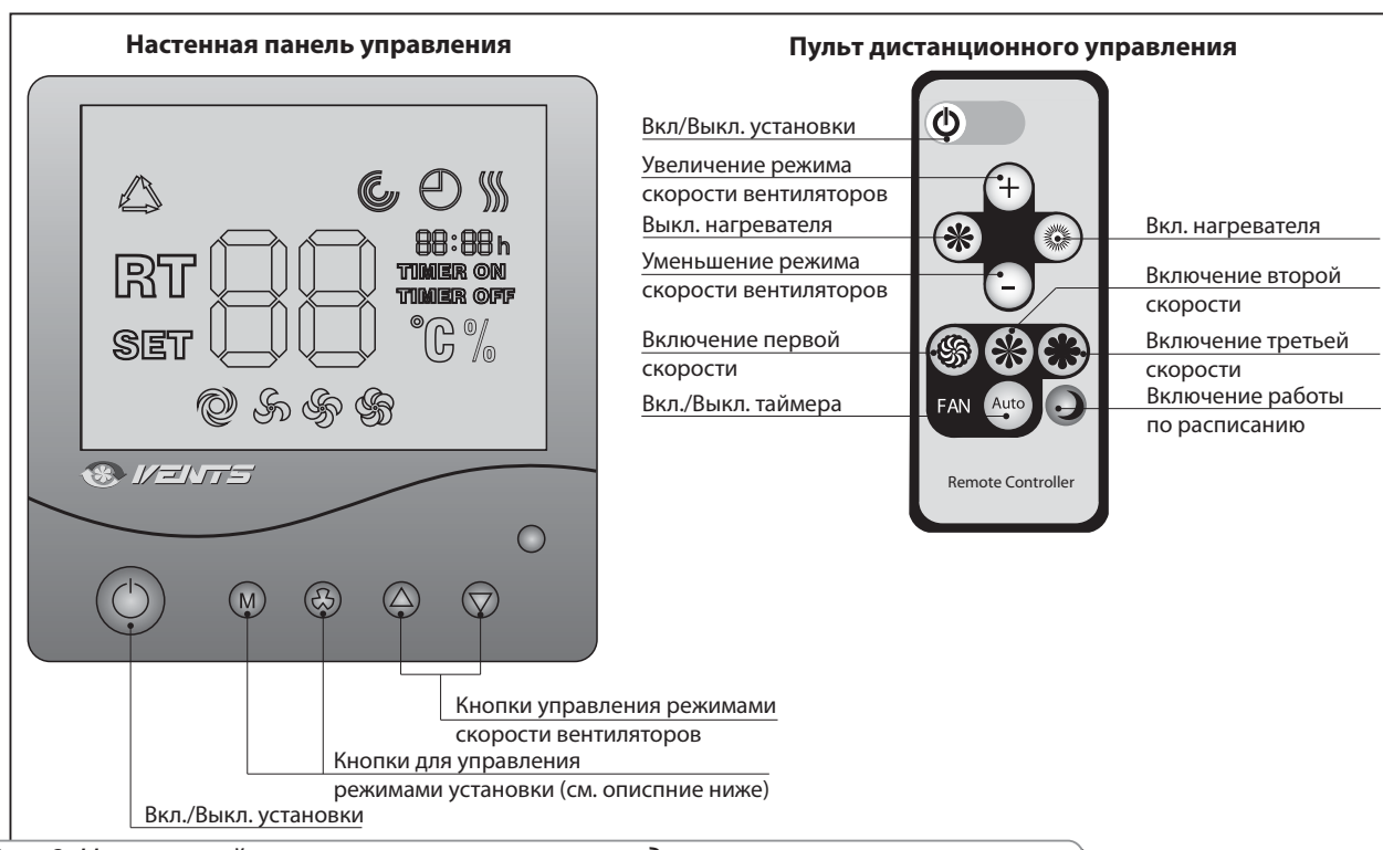
Рис. 8. Настенный пульт управления и пульт дистанционного управления
