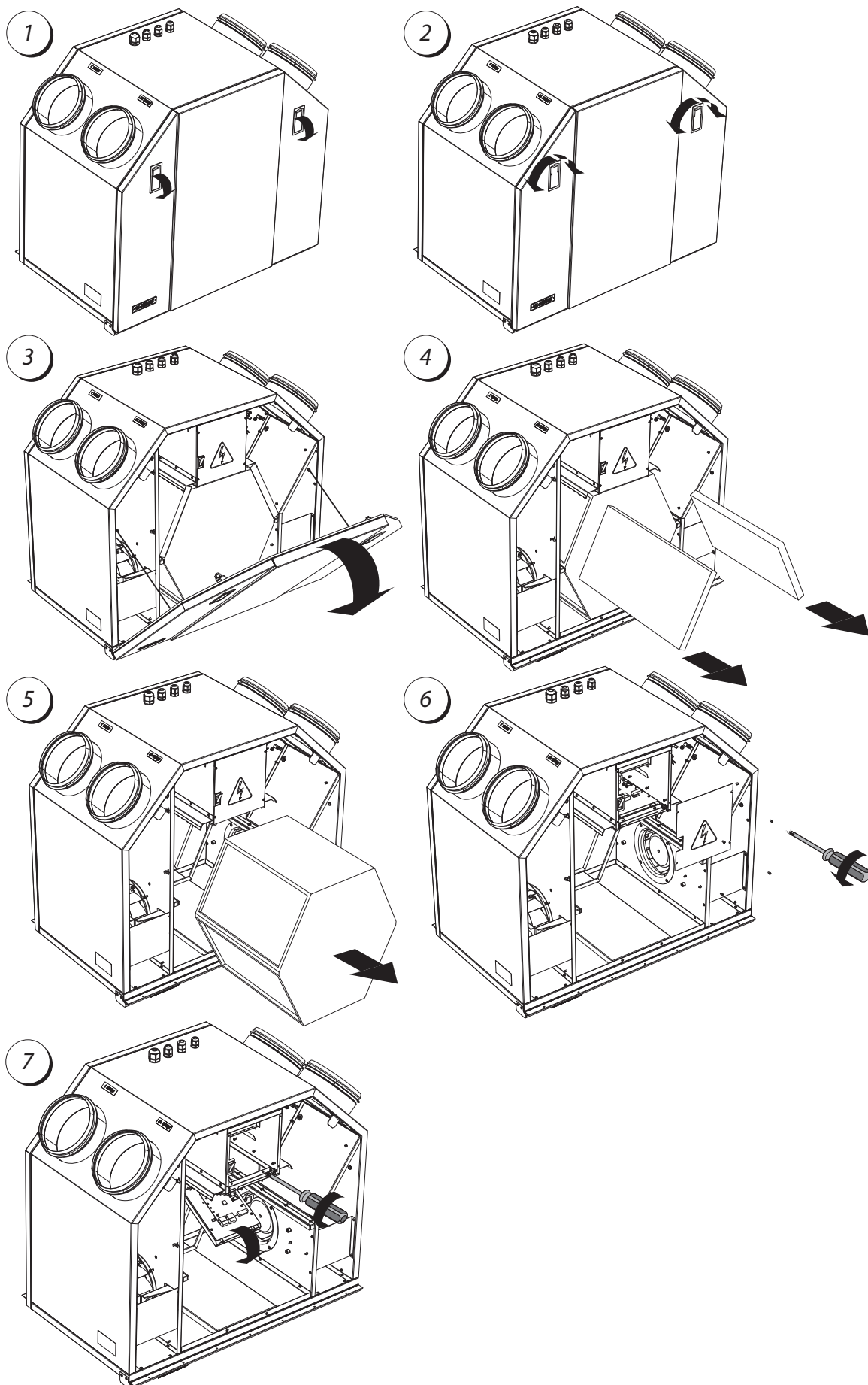
Рис. 18. Обслуживание блока управления
