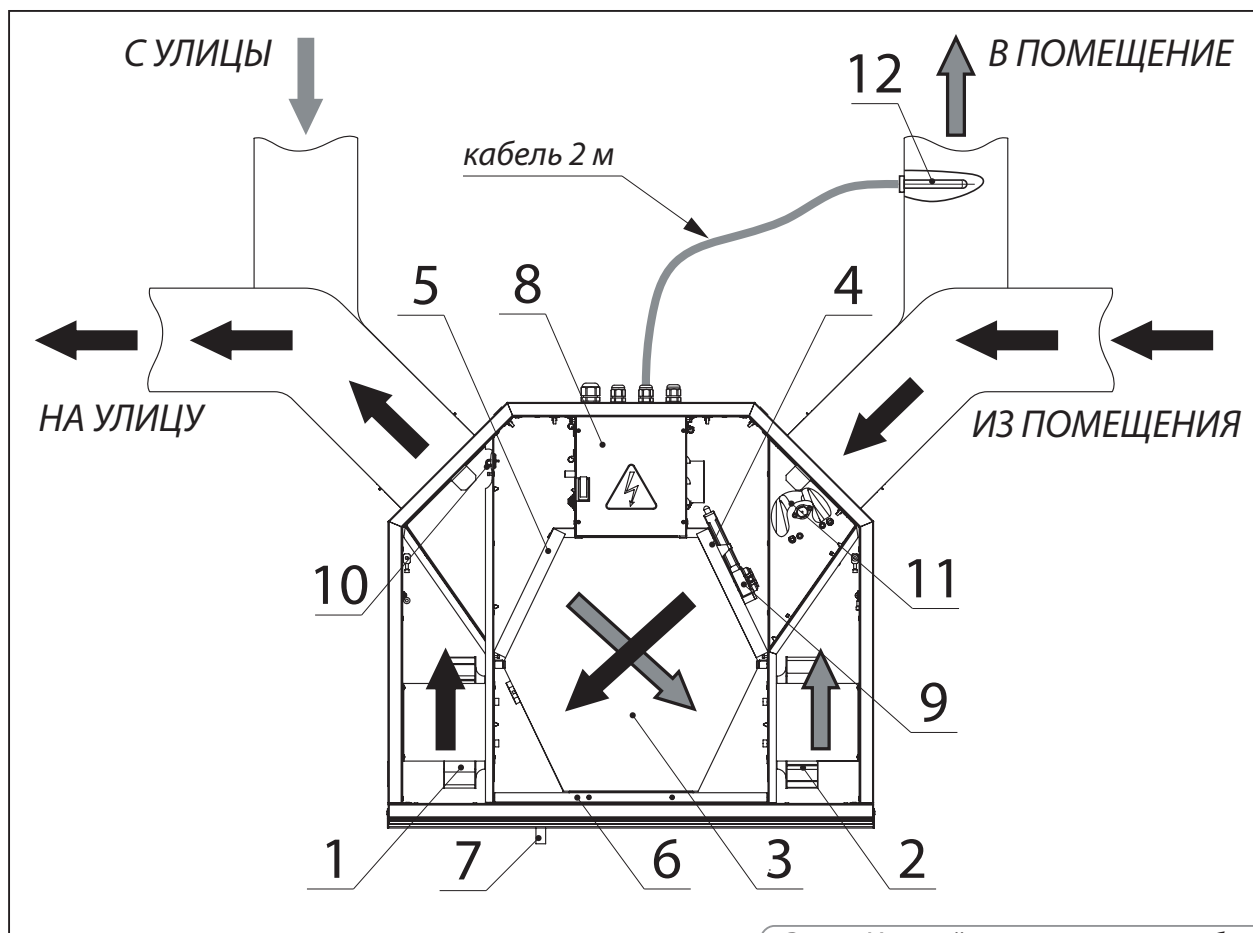
Рис. 2. Устройство и принцип работы
