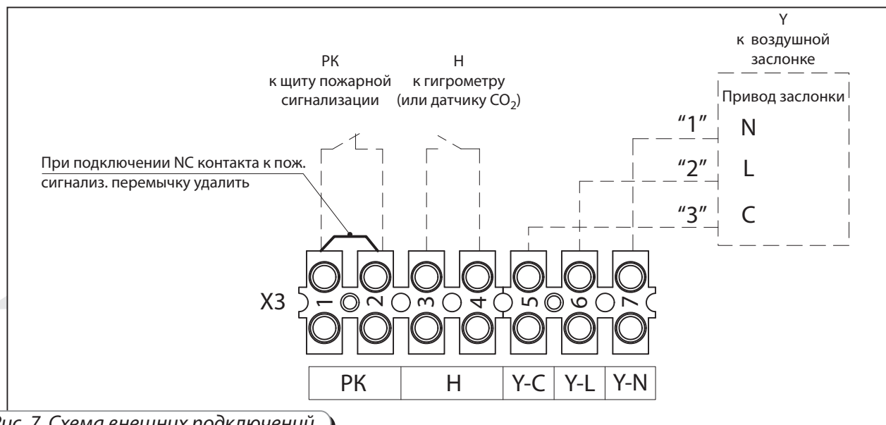
Рис. 7. Схема внешних подключений
