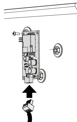
Датчик CO 2
