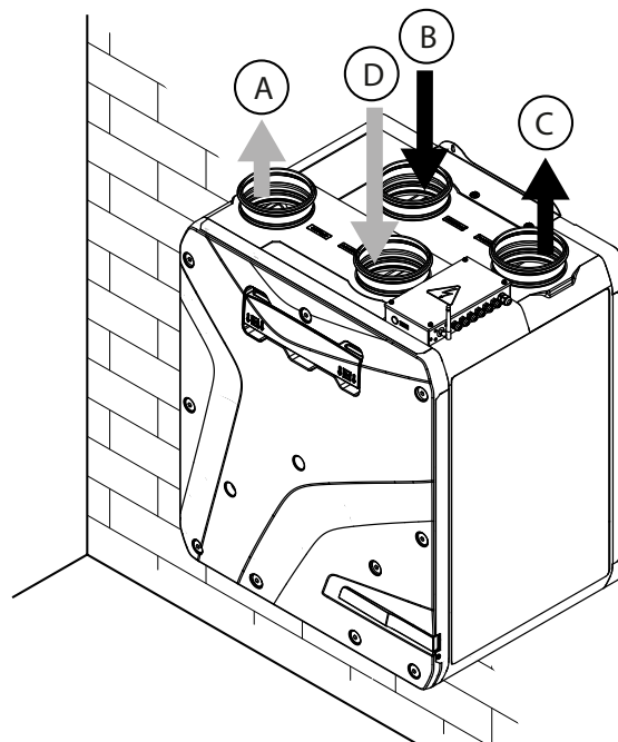
Enave(-T) 350/351/550 V R
