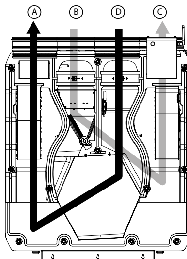
Enave(-T) 350/351/550 V R
